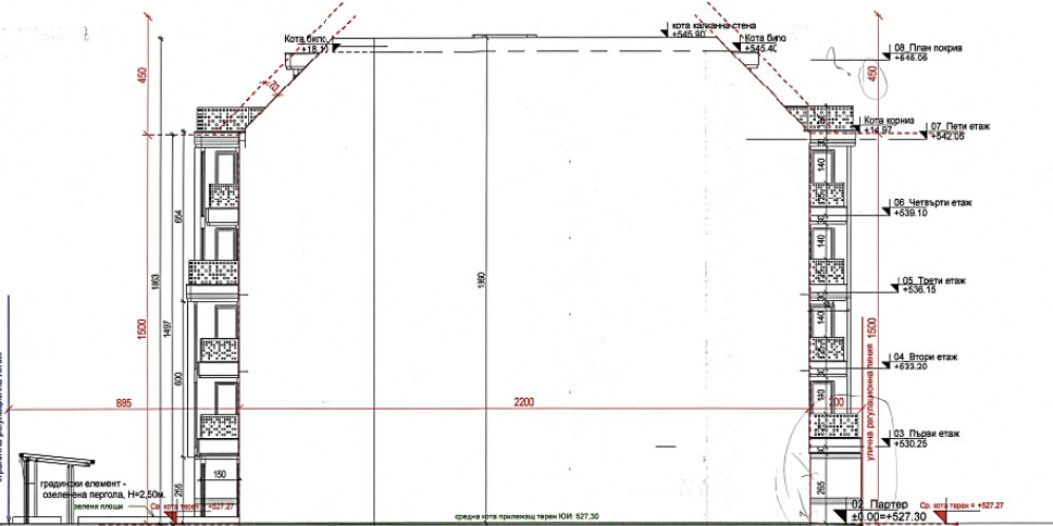
ФАСАДА ЮГОИЗТОК - СВЪРЗАНО ЗАСТРОЯВАНЕ
