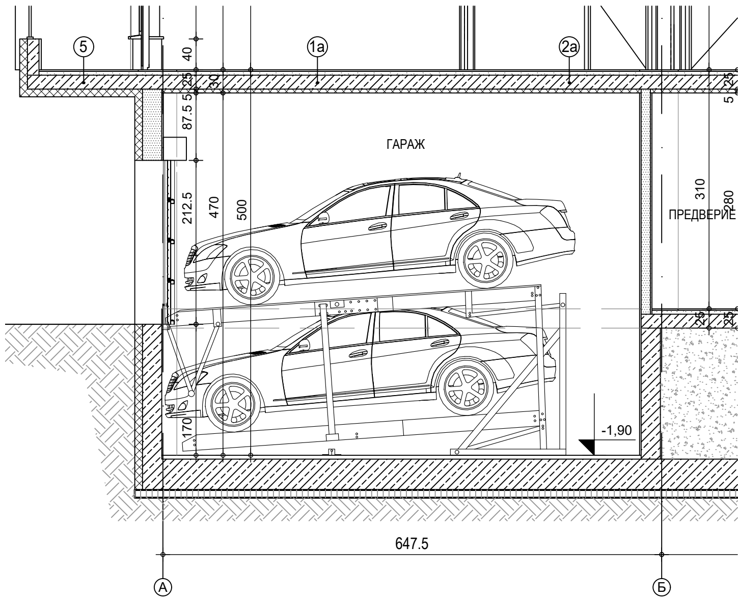
РАЗРЕЗ ГАРАЖ М 1:50
