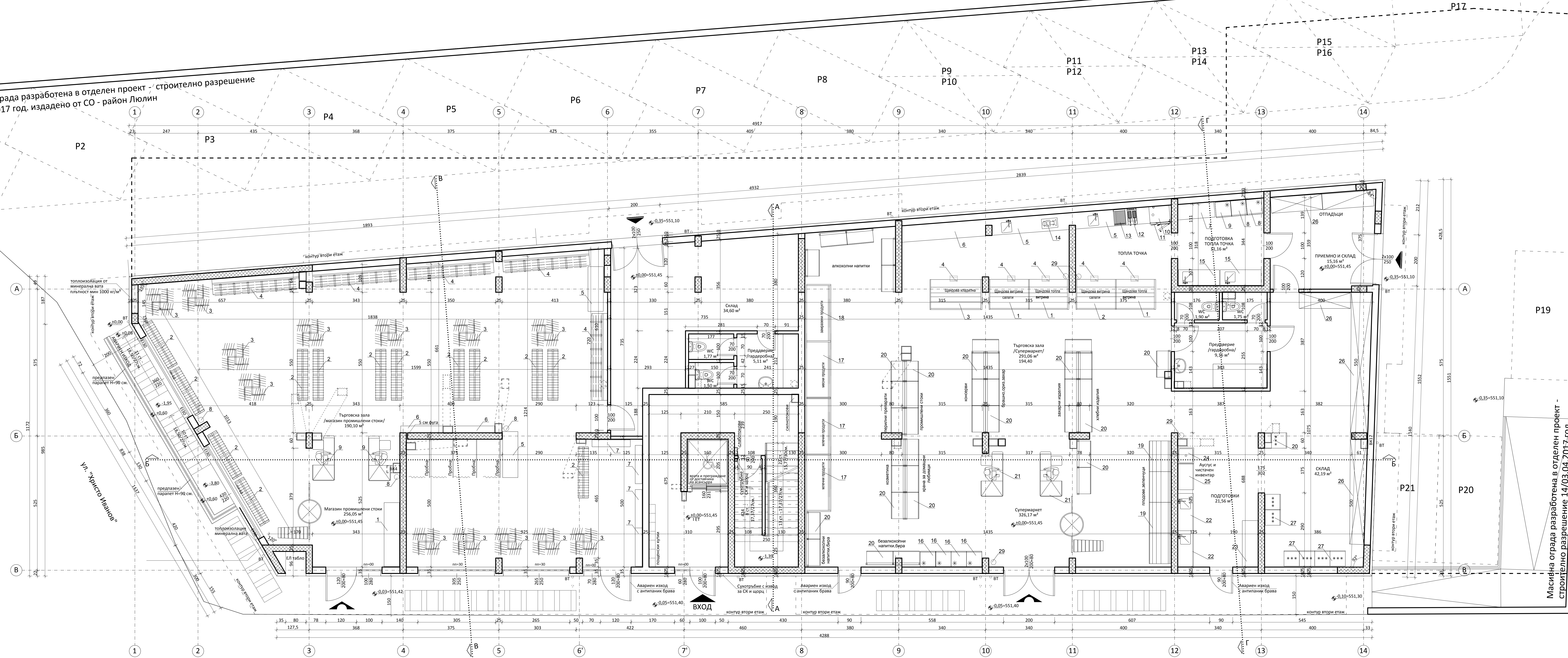
РАЗПРЕДЕЛЕНИЕ НА КОТА ±0.00 M = 1:50
