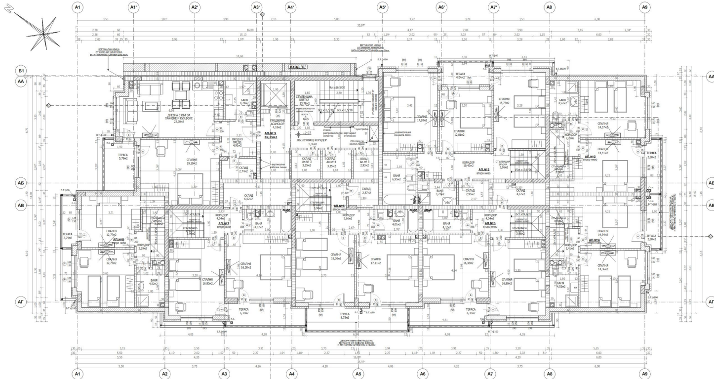
РАЗПРЕДЕЛЕНИЕ НА ВТОРИ ЕТАЖ ВХОД "А" - КОТА - ±2.97 M 1:50
