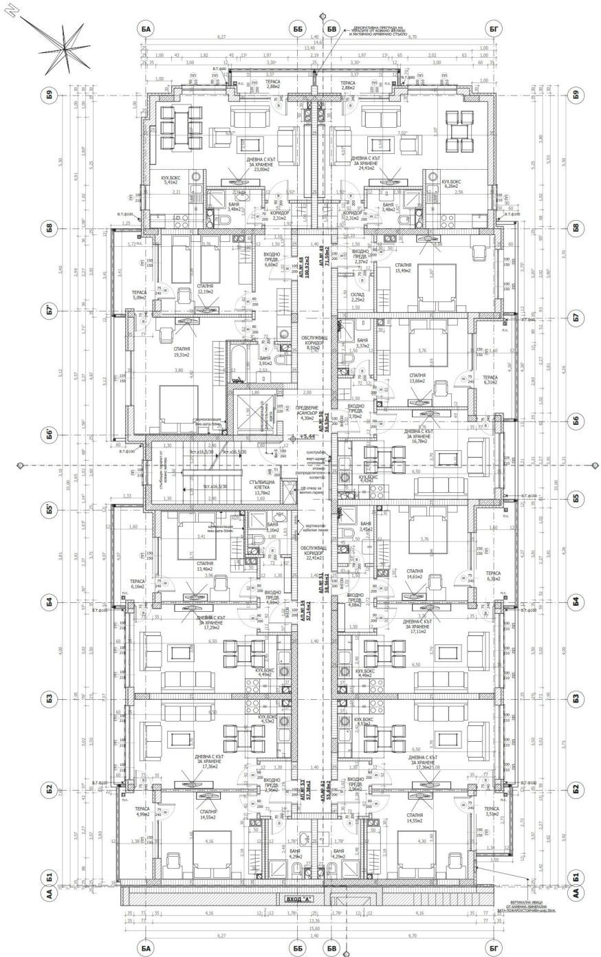
РАЗПРЕДЕЛЕНИЕ НА ТРЕТИ ЕТАЖ ВХОД "Б" - "КОТА" - +5.44" М 1:50
