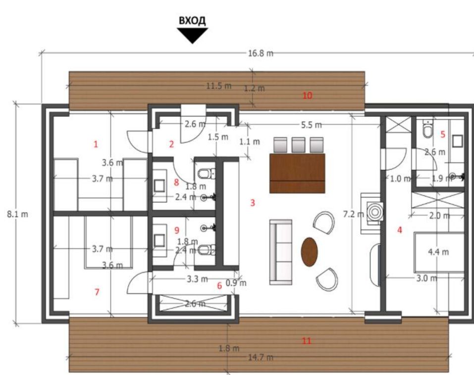
РАЗПРЕДЕЛЕНИЕ ±0.00
