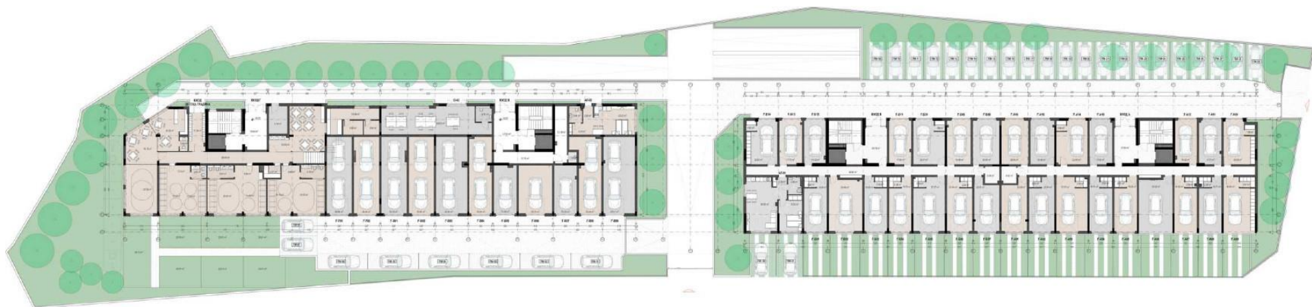
СЕКЦИЯ Г РАЗРЕДЕНИЕ - ПРИЗЕМ ЕТАЖ (М 1:125)
